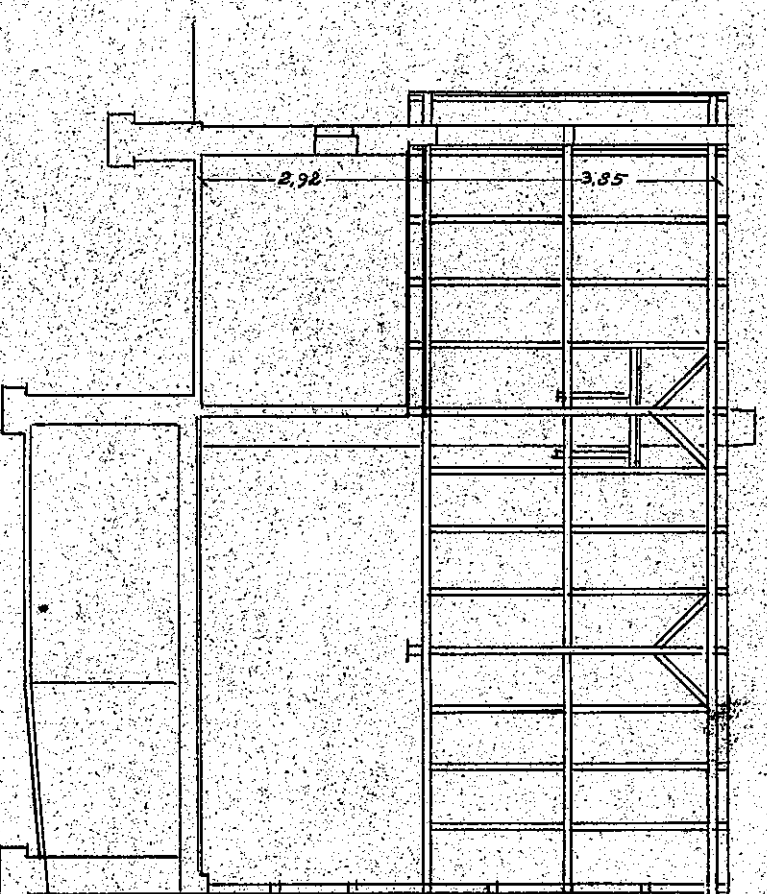
SCHNITT C-D
