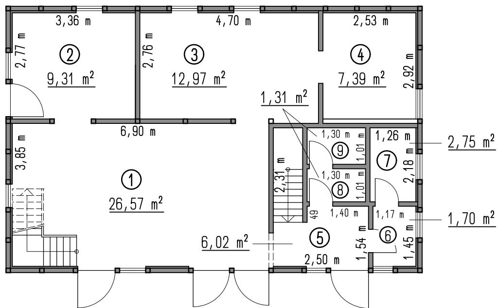
Erdgeschoss
